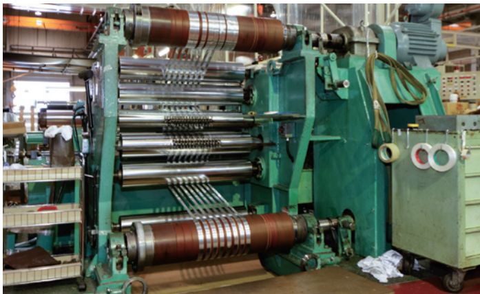
薄板スリッターライン
